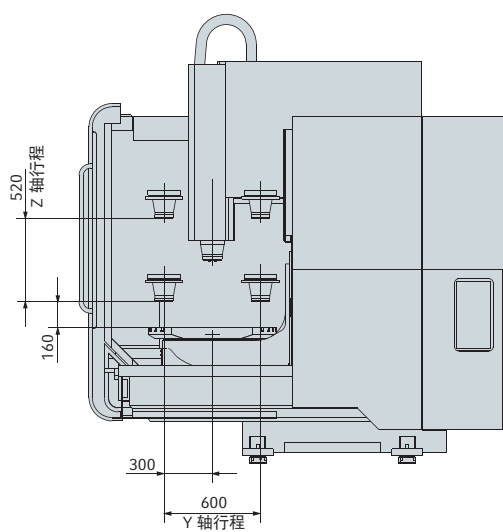
侧视图
