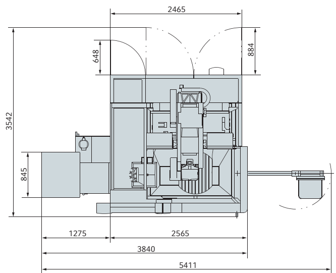
俯视图
