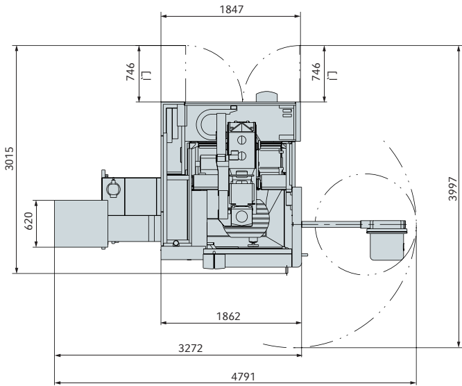
俯视图
