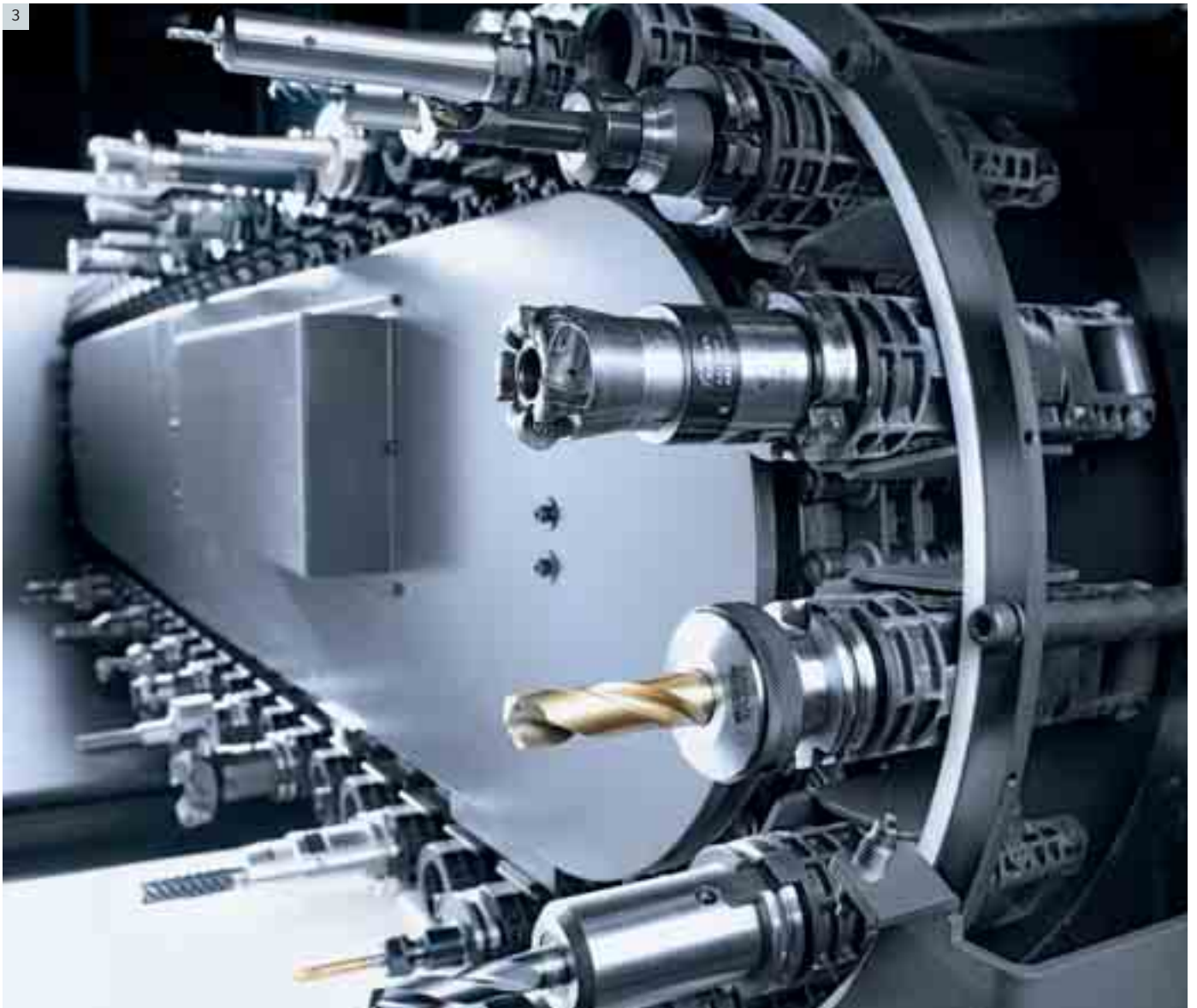
1|1 带 16 刀位和拾取式换刀功能的刀库 |2| 带托盘装卸装置的加工空间 1|3| 带装夹辅助的 30 或 60 刀位的刀库
