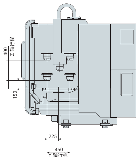
侧视图
