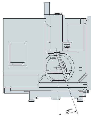
正视图
