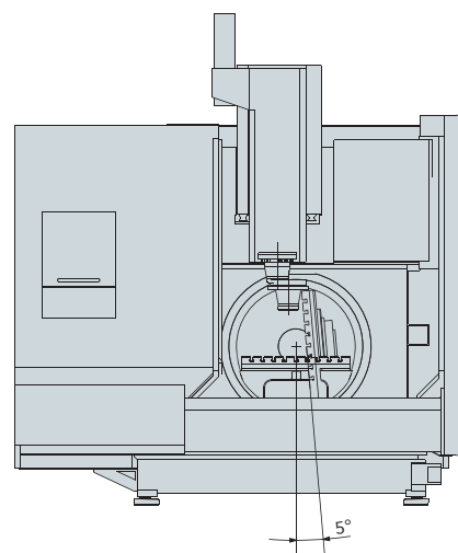
正视图
